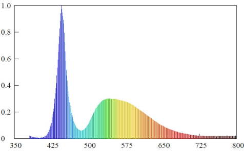
Spectroradiometric Parameters
